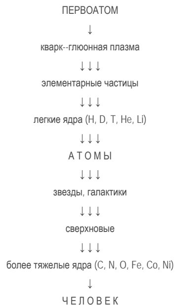
Рис. 1. Схема эволюции Метагалактики от Первоатома до появления Человека.
