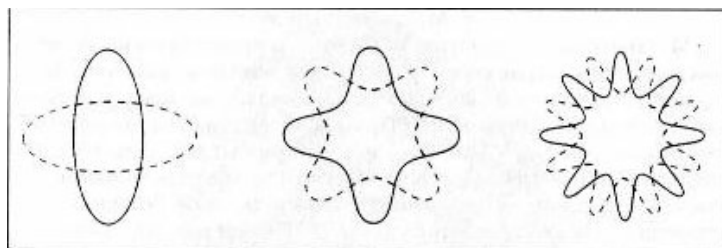
Рис. 4. Моды колебаний суперструн и элементарные частицы, по Б.Грину [14, с. 101].
