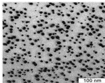
Рис. 2. Электронная микрофотография наночастиц серебра.
