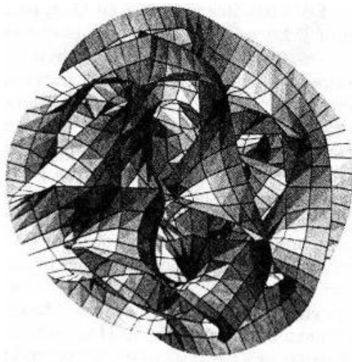
Рис. 5. Дополнительные (свёрнутые) пространственные измерения в теории суперструн (по Б.Грину [14, с. 142]).
