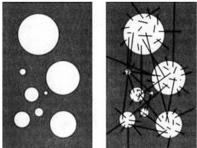
Рис. 3. Модели Большой Вселенной — без тоннелей (слева) и с тоннелями (справа). Так представляют топологию «кротовых нор» акад. Н.С.Кардашев и его коллеги [3-4].
