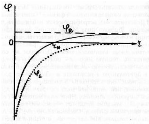
Рис. 7. Зависимость гравитационного потенциала от расстояния с учётом постоянного положительного поля.
