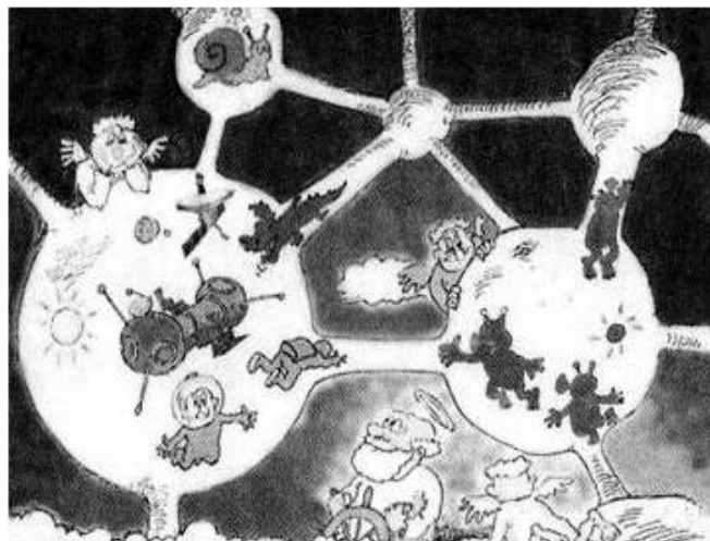
Рис. 4. Большая Вселенная: «пузырьки» и соединяющие их тоннели. Так представляют себе ту же топологию некоторые сотрудники ИКИ РАН [5].
